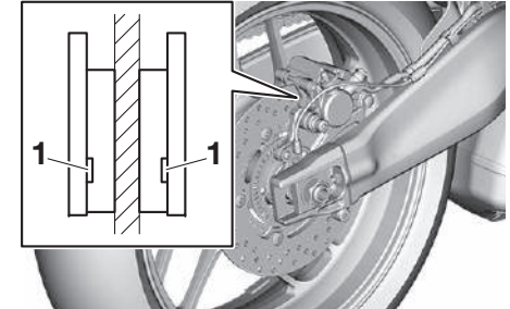
1. Ranura indicadora de desgaste de la pastilla de freno
