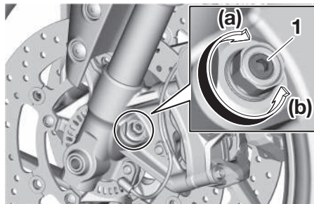
1. Regulador de la amortiguación en compresión lenta
