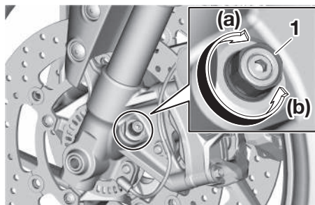
1. Regulador de la amortiguación en compresión rápida
